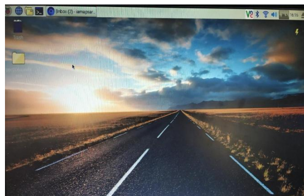
Fig 3: Raspbian OS
